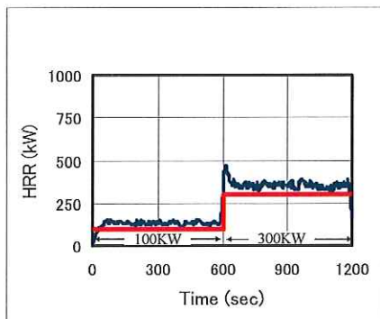
図5 ISO9705 ルームコーナーテストでの フラッシュオーバー現象
