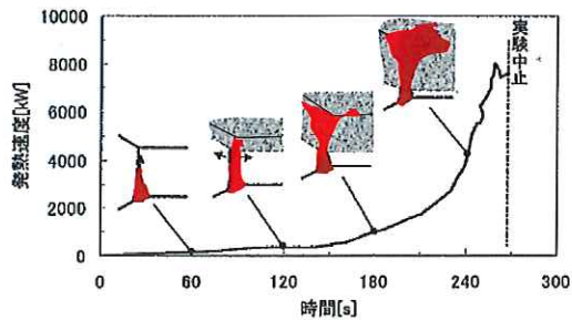
図7-1 ルームコーナー試験における内装材料の発熱速度想定例
