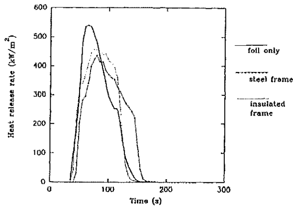
図 13-5 Polystyrene foam
