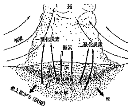
図6 くん焼時の熱と物質の流れ
