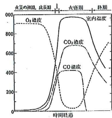
図 8-2 火災時の室内の温度、濃度の変化
