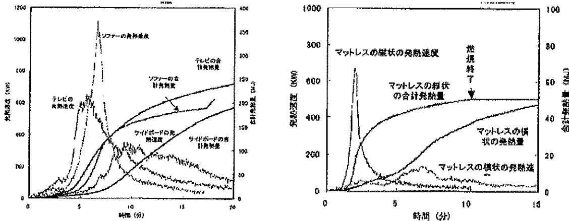
図 13-1 各種収納可燃物の発熱速度 (閉鎖空間)
