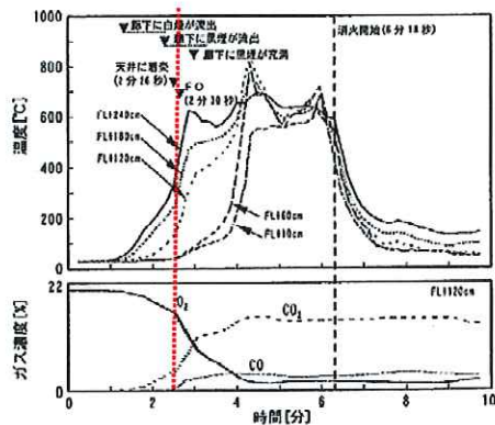
図8-1 ホテル客室の火災実験における温度とガス濃度の変化
