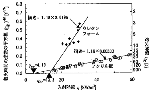
図10-2 ウレタンフォームの着火時間
