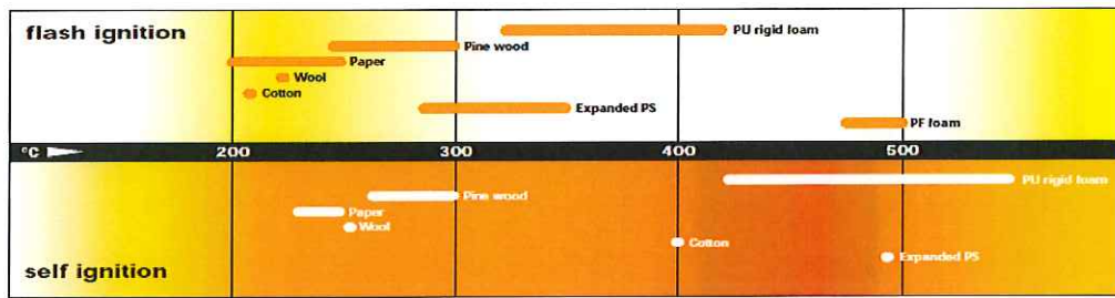
図 11 各種材料の着火温度
