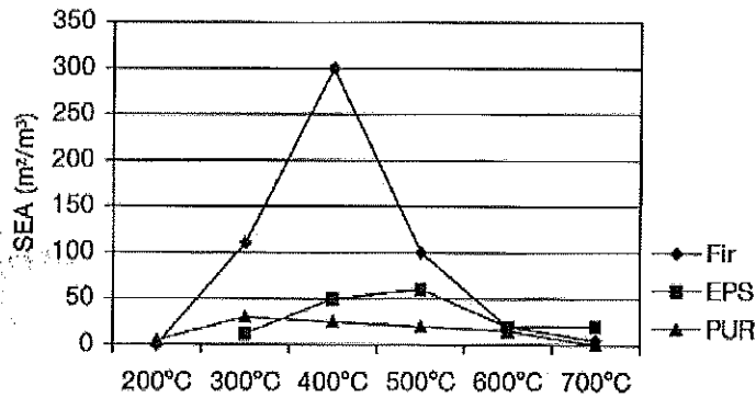
図 23-4 発煙量に対する加熱温度の影響
