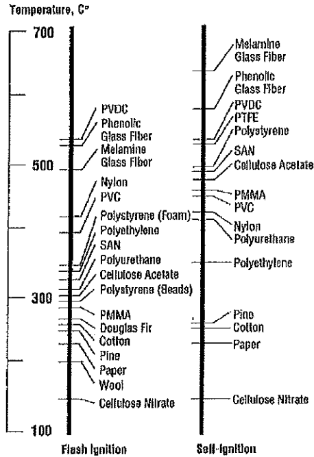
図 10-1 各種プラスチック材料の発火温度
