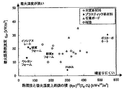
図10-3 各種材料の着火特性値
